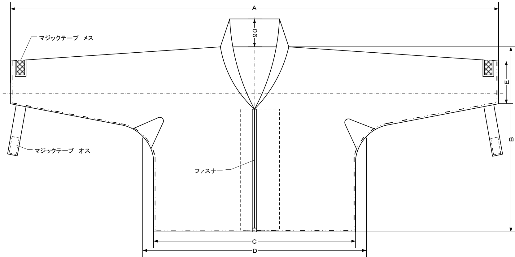
標準寸法表
